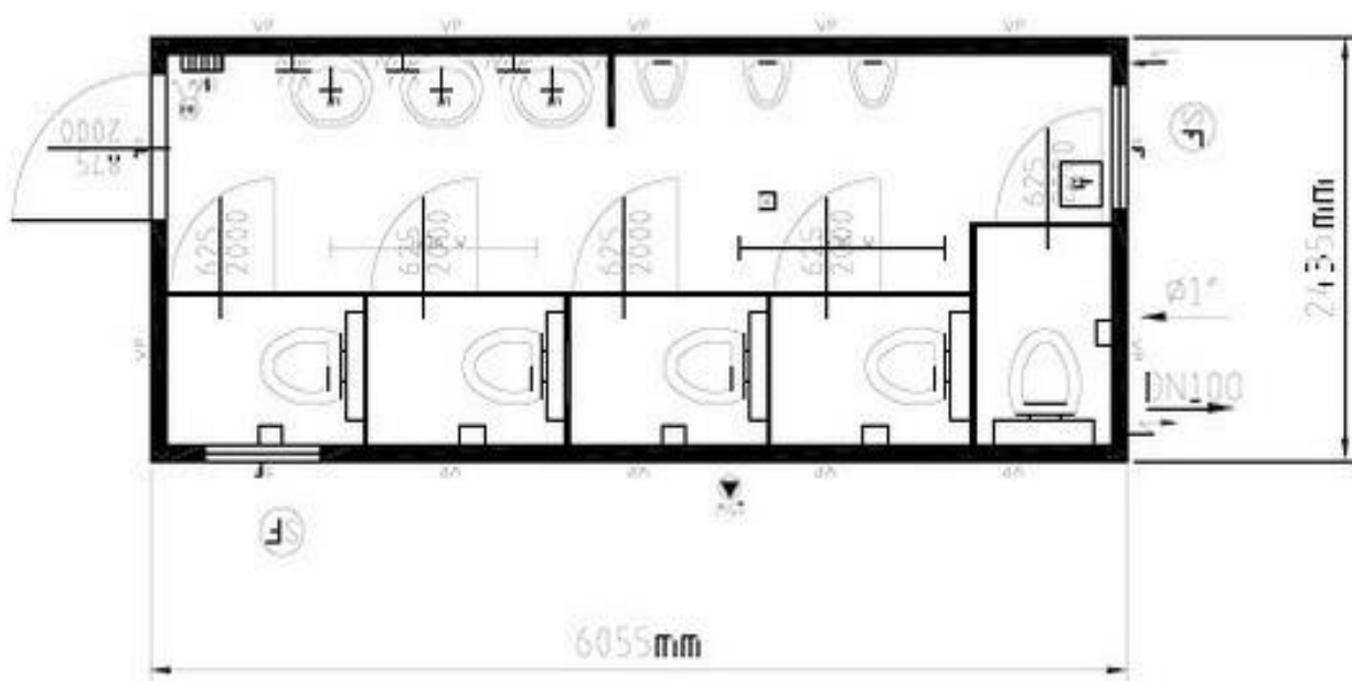
Схематичний план громадської вбиральні модульного типу
