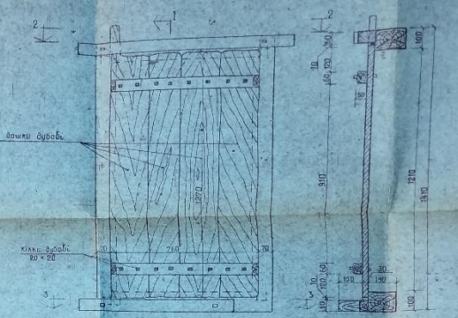
ДІБЕРІ НА БІГНАХ З ПІДВАЛІСЬКОЮ СІМ'ЯНИНОЮ ВЗД. 3-3 ПРИБЛИЖНО М. 1:10
